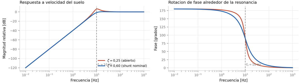
Figura 1: Modelo nominal del SM-24 referido a velocidad del suelo. La carga resistiva aumenta el amortiguamiento y aplanan la resonancia, pero no elimina la caída de segundo orden por debajo de 10 Hz. Figura generada con los parámetros de la hoja de datos.
